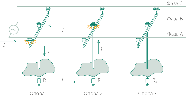
Схема 4. Схема установки разрядников ИРШФМК-10(20) на ВЛ
