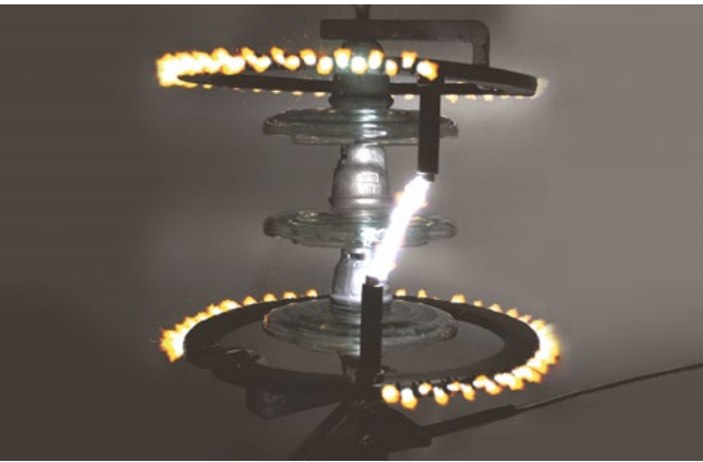
Фото. 5. РМКЭ-35 в процессе гашения
