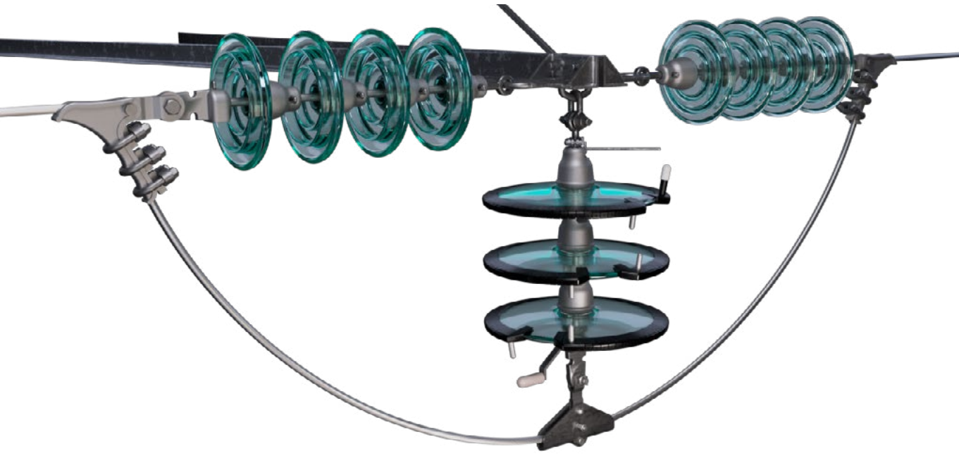
Рис. 23. Установка ГИРМК-35 на анкерно-угловой опоре
