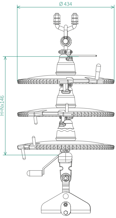
Габаритные размеры ГИРМК-35 N - количество ИРМК в гирлянде
