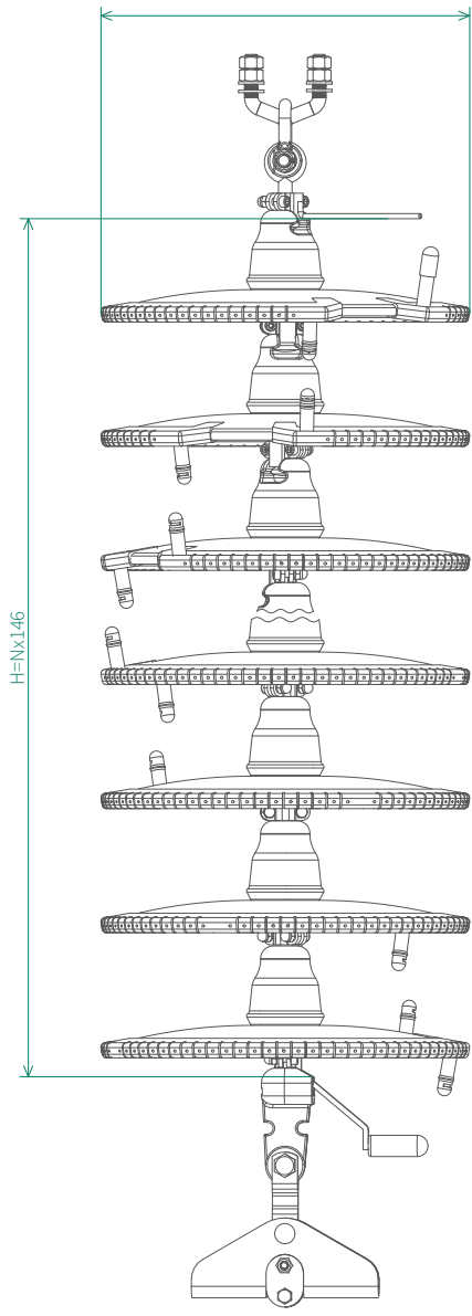
Габаритные размеры ГИРМК-110 N - количество ИРМК в гирлянде
