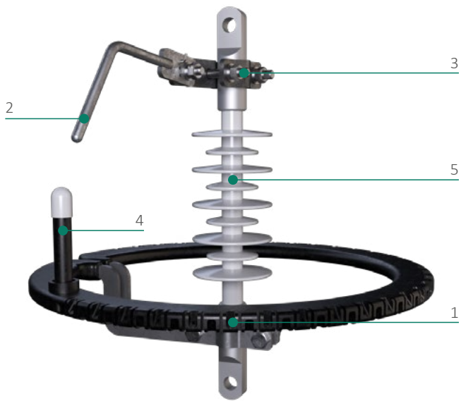
Рис. 13. Общий вид разрядника РМКЭ-20 в стандартной комплектации
