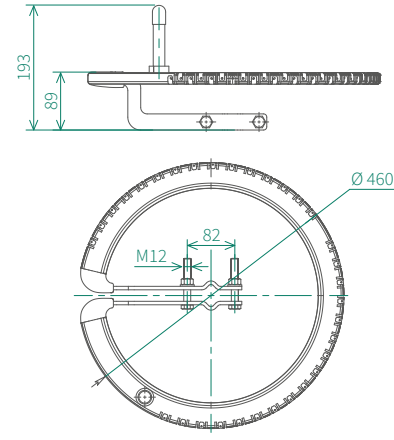
Габаритные размеры РМКЭ-20, РМКЭ-35
