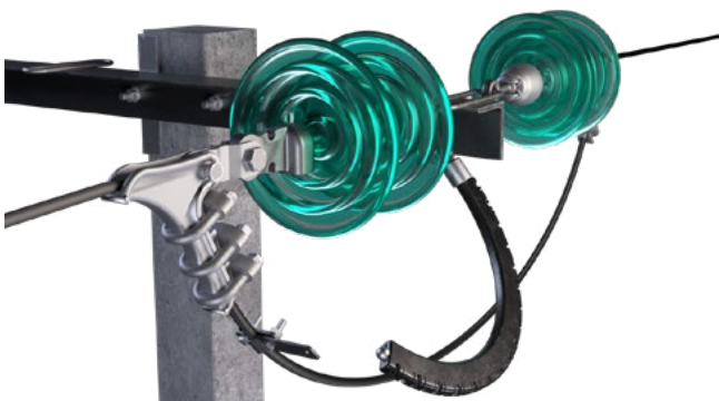
Рис. 9. Установка РМКЭ-10 совместно с натяжной стеклянной изоляцией
