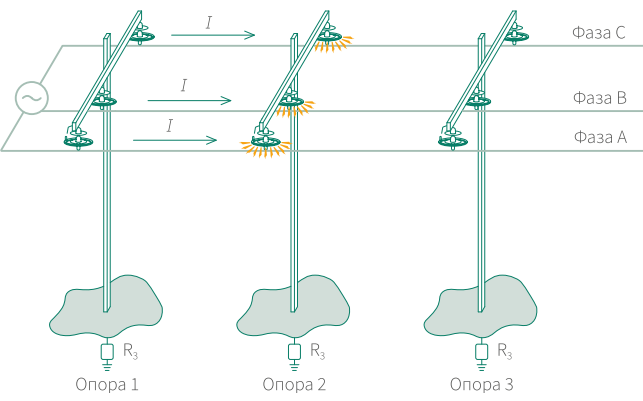
Схема 6. Схема установки разрядников РМКЭ-20 на ВЛ для защиты от отключений при ПУМ
