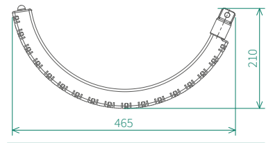
Габаритные размеры РМКЭ-10
