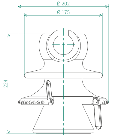
Габаритные размеры ИРШФМК-10(20)
