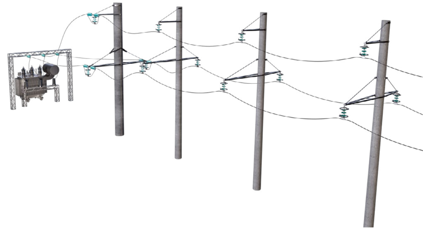
Рис. 29. Защита подхода ВЛ 35 кВ к подстанциям
