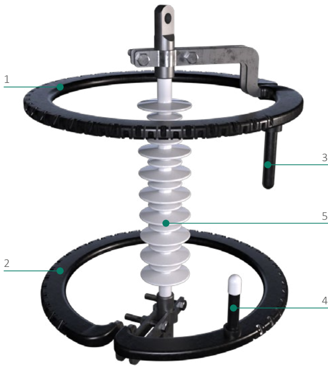
Рис. 17. Общий вид разрядника РМКЭ-35 в стандартной комплектации
