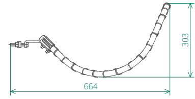
Габаритные размеры РДИП-10
