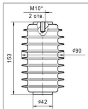
ОПН-П 3,3 КС
